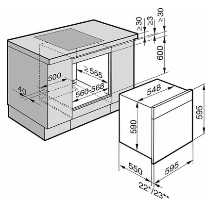
DGC 6000, CLST (Skizze)
