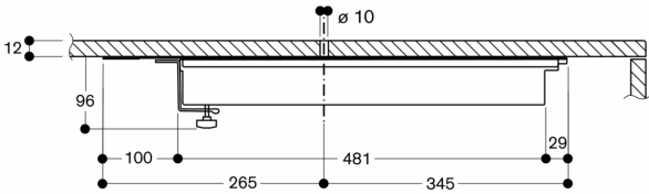
Longitudinal section
