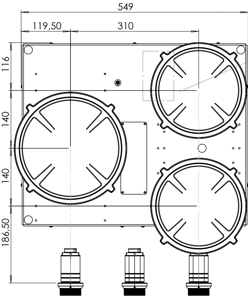
Bovenaanzicht / Top view
